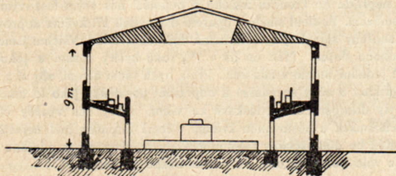
PŘÍČNÍ ŘEZ
